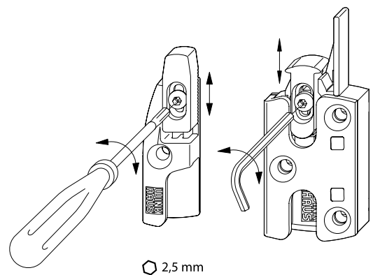
Rahmenteil DFE/TFE
